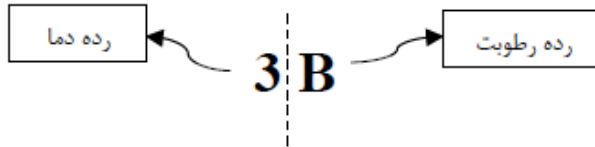
شکل ۱۹-۳-۱: نحوه نمایش تقسیم‌بندی اقلیم‌ها
